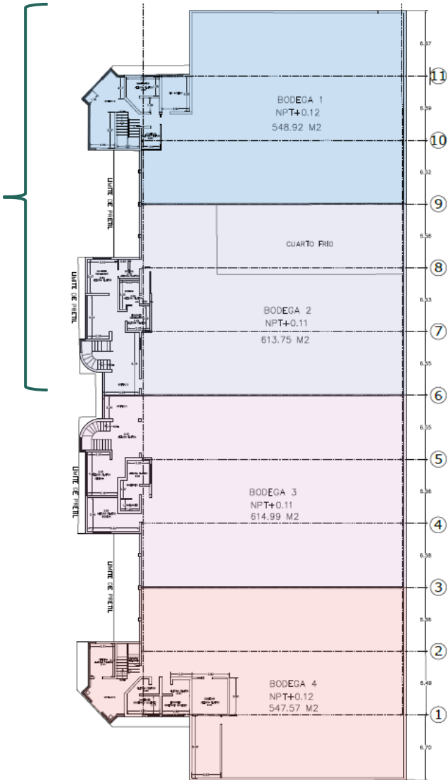
PLANTA BAJA
